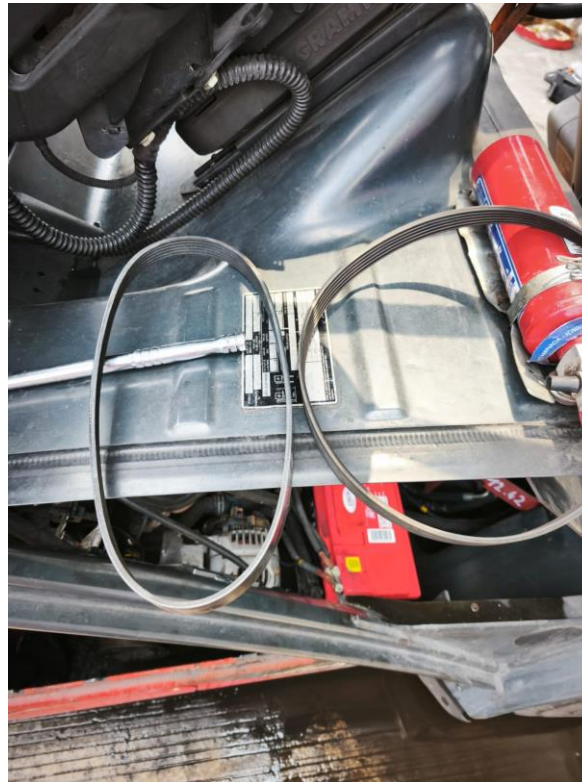
REEMPLAZO DE BANDA DE ALTERNADOR
