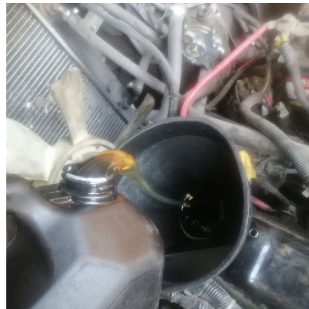
REEMPLAZO DE ACEITE DE MOTOR
