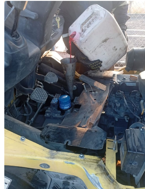
REEMPLAZO DE ACEITE DE TRANSMISION
