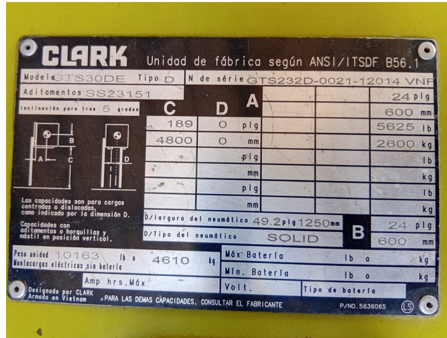
PLACA DE DATOS DEL MONTACARGAS
