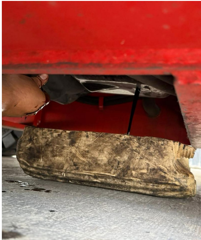
DRENADO DE ACEITE DE MOTOR
