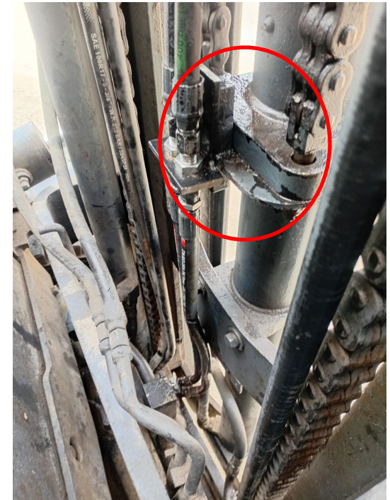
INSTALACIÓN DE 2 PASA MUROS PARA MANGUERA VIAJERA
